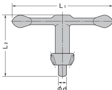
新型(一体型)
