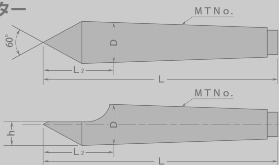
仕様寸法表 (単位:mm)
